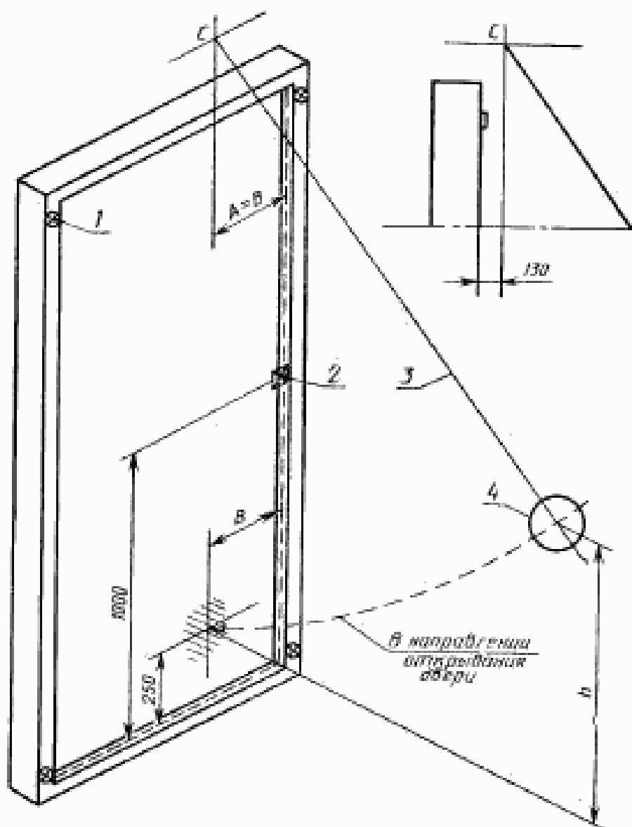
1 — пружин; 2 — запирающий прибор или ограничитель; 3 — гибкая нить; 4 — неупругое тело (груз). B = \frac{1}{2} ширины полотна, но не более 300 мм.
