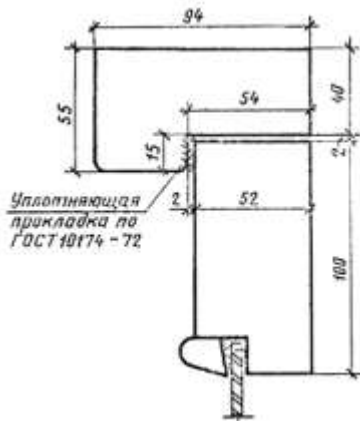
Сечение В2
