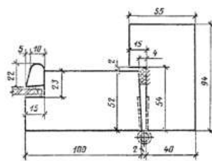
Сечение В3
