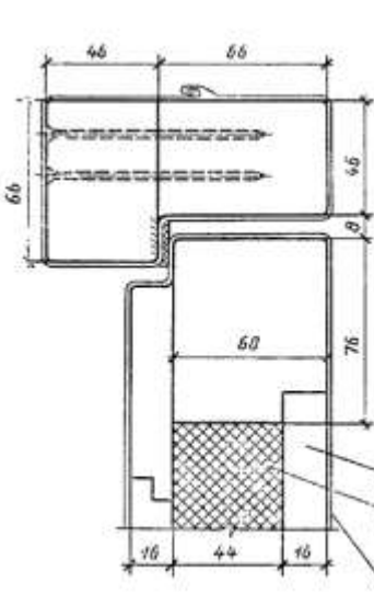
Сечение Ж1
