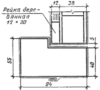
Сечение Е2
