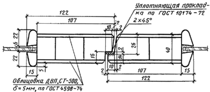
Сечение А6
