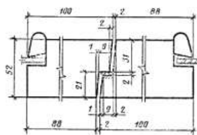
Сечение В4
