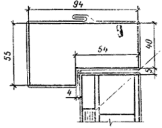
Сечение Е1
